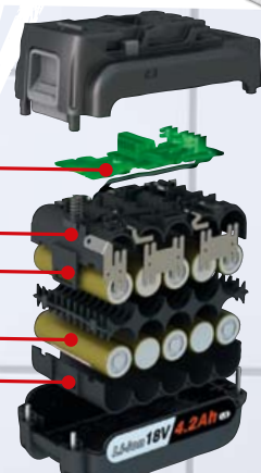
Afgebeelde batterij : EY9L51B 18V / 4,2Ah
