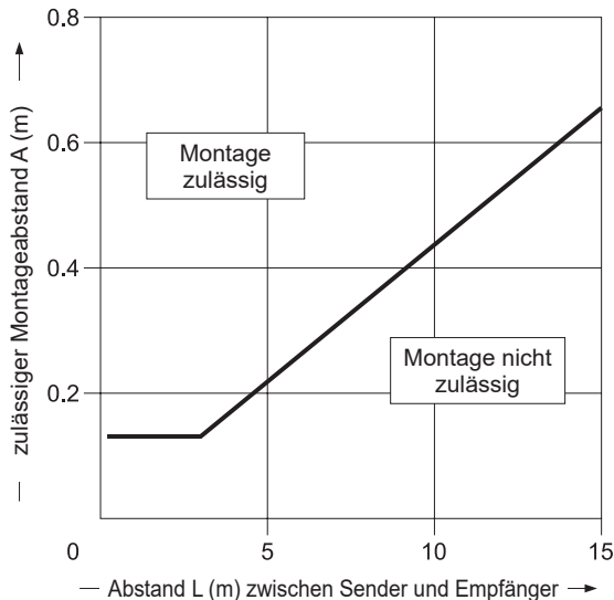
Zulässiger Montageabstand zu reflektierender Fläche
