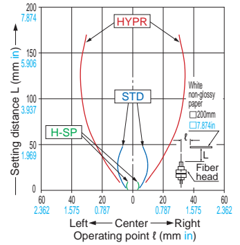
FD-EG30
