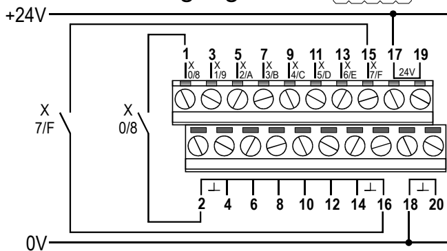
Eingänge NPN
