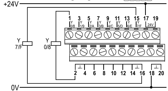
Ausgänge PNP
