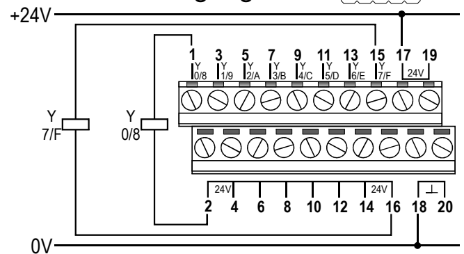
Ausgänge NPN
