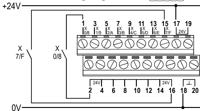
Eingänge PNP
